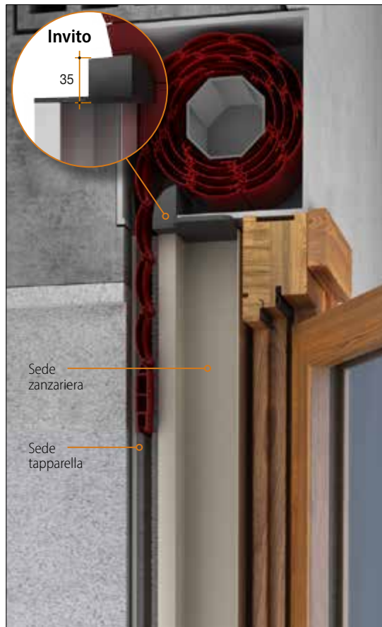
Esempio di installazione Guida Tapparella da 90mm
