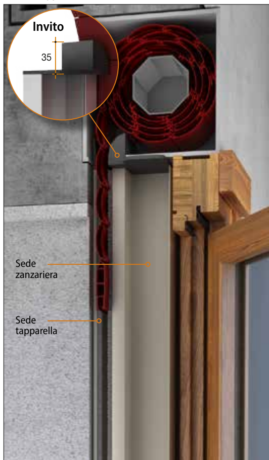
Esempio di installazione Guida Tapparella da 90mm
