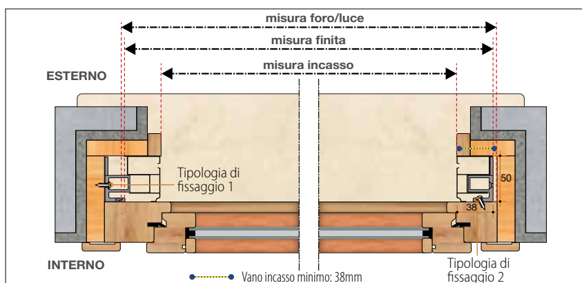
Sezione orizzontale
