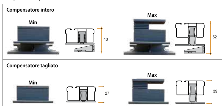
Compensazioni possibili
