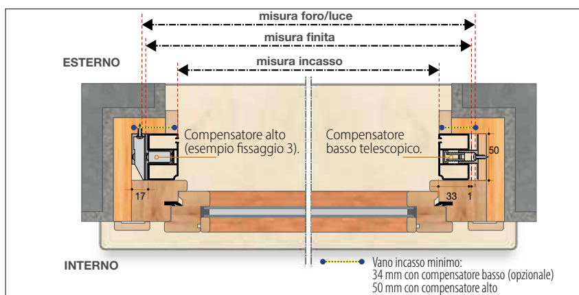
Sezione orizzontale
