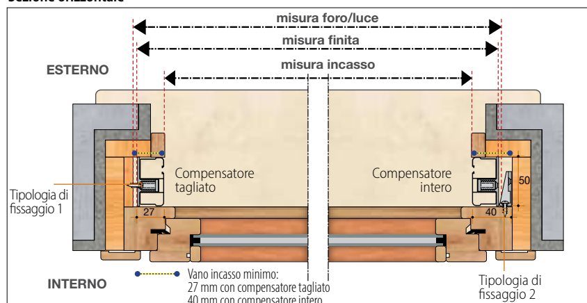
Sezione orizzontale
