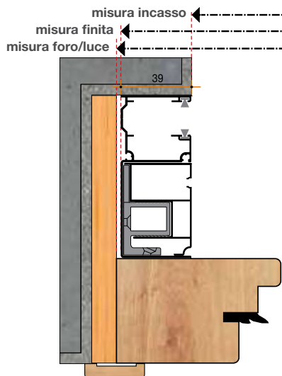
Esempio di installazione Guida Tapparella da 90mm
