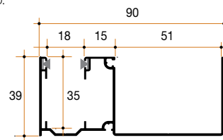
tipologia di fissaggio 1
