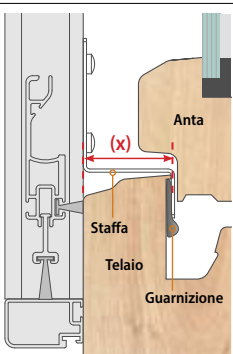
Serramento non planare
