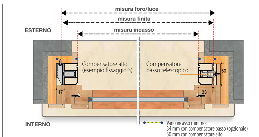
Sezione orizzontale
