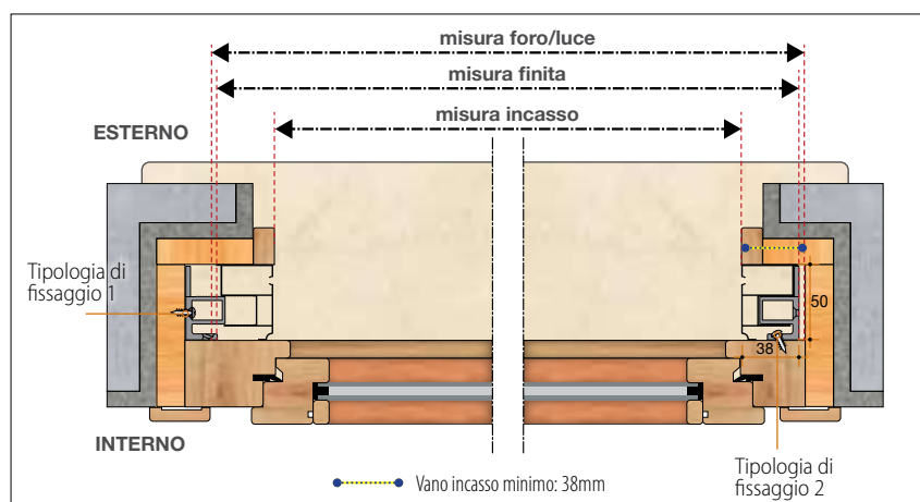
Sezione orizzontale
