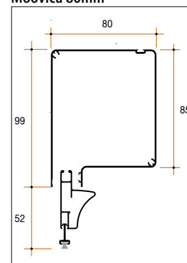
Ingombro gruppo Cassonetto Moovica 80mm
