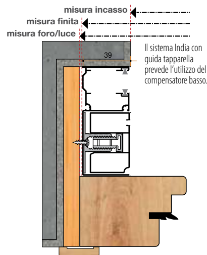
Esempio di installazione Guida Tapparella da 90mm
