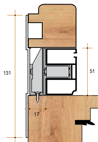
Esempio con compensatore alto.
