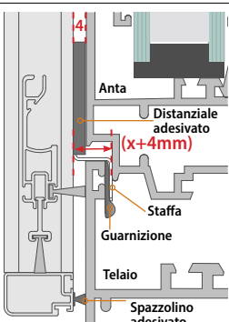
Serramento planare
