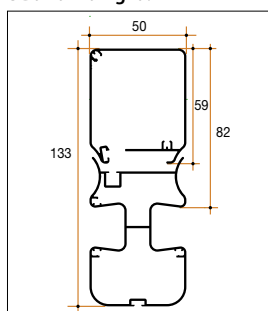
Ingombro Cassonetto e Barra maniglia.
