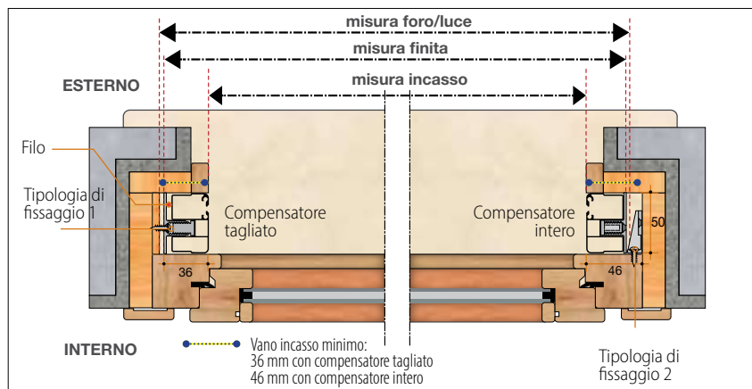
Compensazioni possibili
