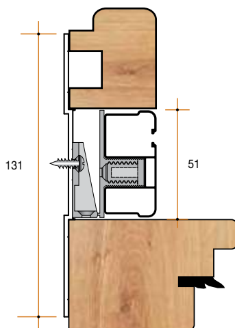
Esempio con guida e compensatore
