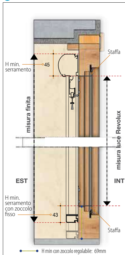
Serramento planare
