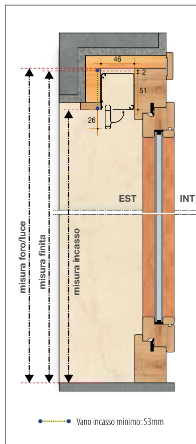
Sezione verticale
