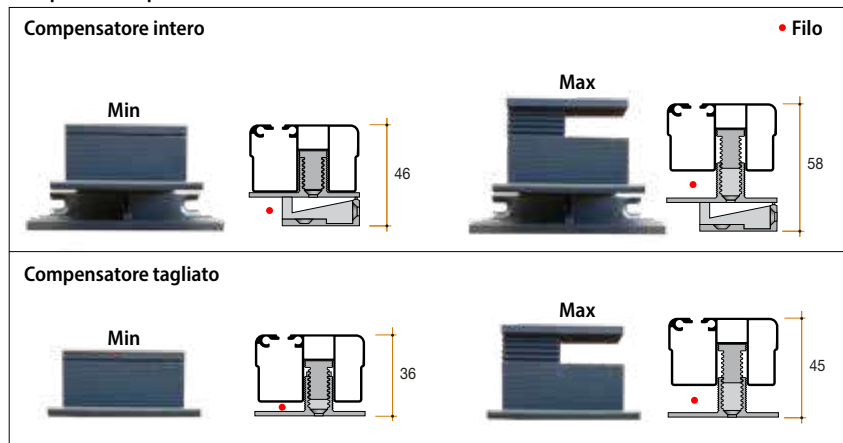
Compensazioni possibili
