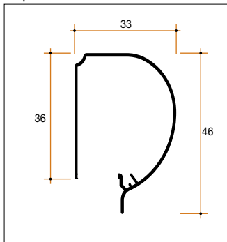
Ingombri
