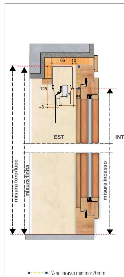
Sezione verticale
