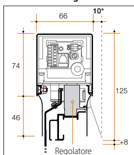
Carter Motore e guida
