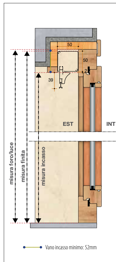
Sezione verticale
