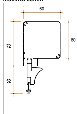
Ingombro gruppo Cassonetto Moovica 60mm
