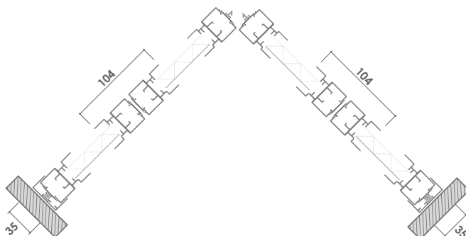
SEZIONE ORIZZONTALE 3 ANTE A SEGUIRE ANGOLARE
