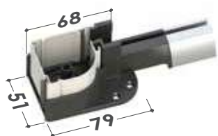
■ Cassonetto da 45 Testate inferiori
