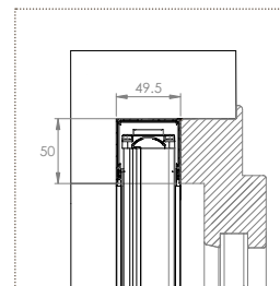
■ BORA INCAS SR MIDI
