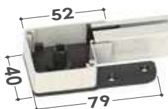
■ Cassonetto da 40 Testate inferiori
