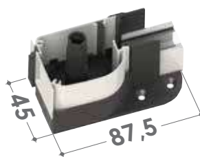
■ Cassonetto da 42 Testate inferiori
