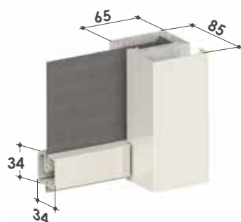
■ Guida e compensatore plus da 85
