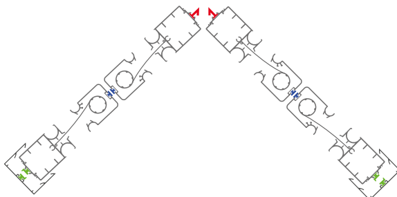
ANTA TRIPLA A SEGUIRE ANGOLARE
