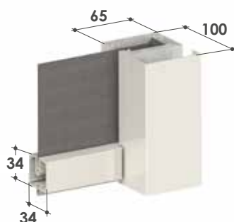
■ Guida e compensatore plus da 100
